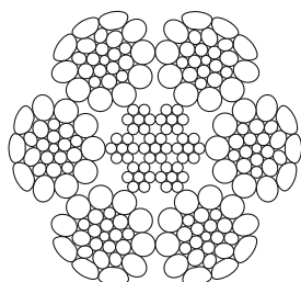
6x26WS+IWRC 205 fili/wires
